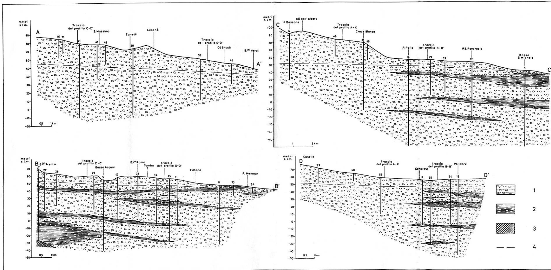
Figura 7 – Sezioni stratigrafiche.
